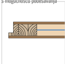
KRILO 46 mm ojačano čeličnim limom
