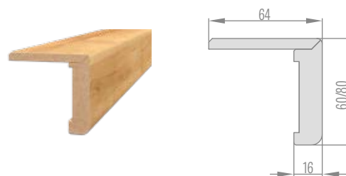
KUTNIK S PRODULJENIM PEROM ZA PODESIVI DOVRATNIK
