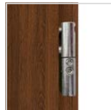
4 PANTI SA SA DVA PINA Ø16 SA 3D PODEŠAVANJEM
