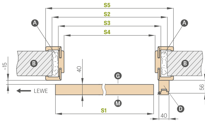
SP1Nz ili SP1Nb (lijeva verzija awers)
